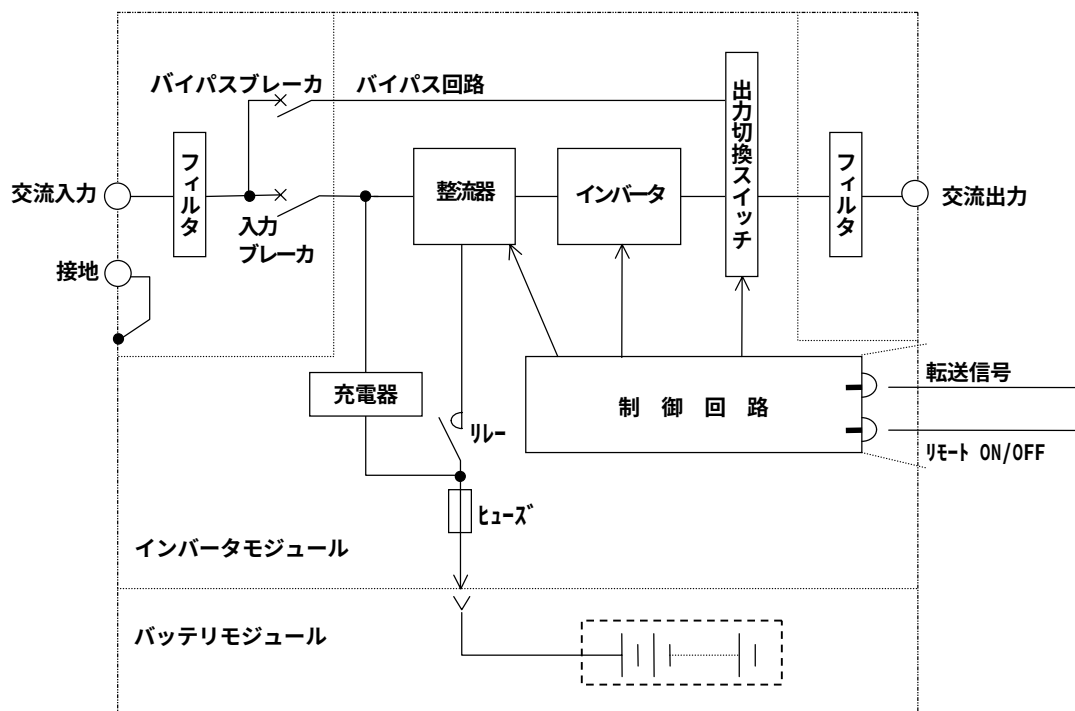
回路系統図
