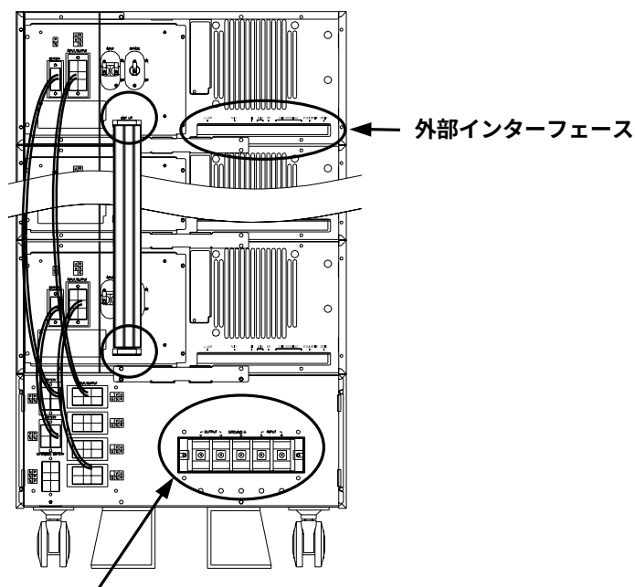
装置裏面
