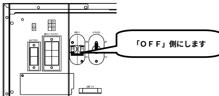
装置裏面
