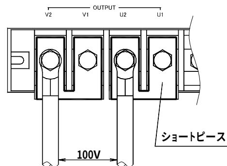
単相2線 100V の場合
