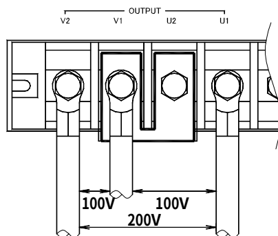
単相3線 100V/200V の場合
