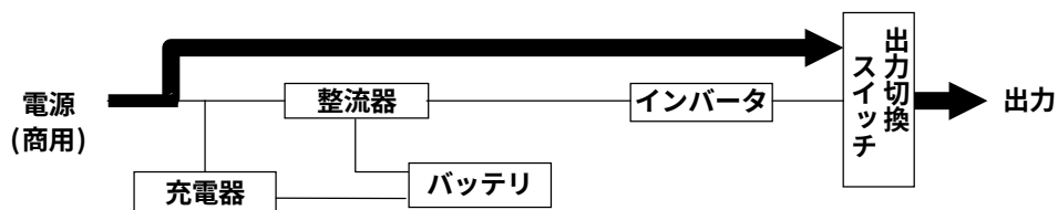
インバータユニット故障時の電力供給経路
