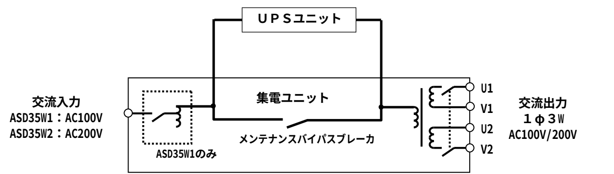
回路系統図
